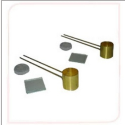
Le-Chatelier Mould
